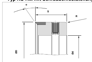
Typ NS-HM mit Schraubenfeststellung
