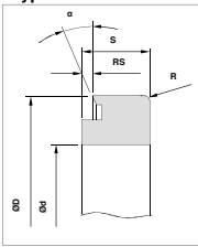
Typ NN ohne Nut
