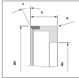
Topfmesser HM
