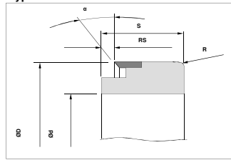
Typ NN-HM ohne Nut
