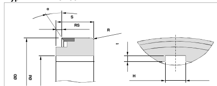
Typ NN-HM mit Nut
