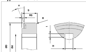
Typ NN mit Nut
